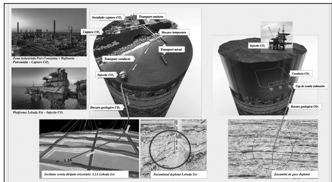
Figura 16. – Prezentarea schematică a modului în care zăcămintele de pe aliniamentul Lebăda pot fi transformate după încheierea ciclului de producție în facilități de stocare a CO 2
