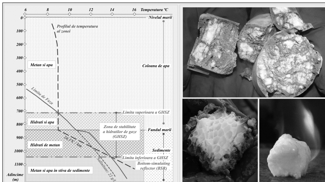
Figura 20. – Diagramă de fază prezentând condițiile de stabilitate a hidraților de metan în sectorul românesc al Mării Negre (cu modificări, după Riboulot et al., 2017). Colaj de fotografii cu eșantioane și fragmente de carote conținând hidrați de metan (sursa: fototeca US Geological Survey).
