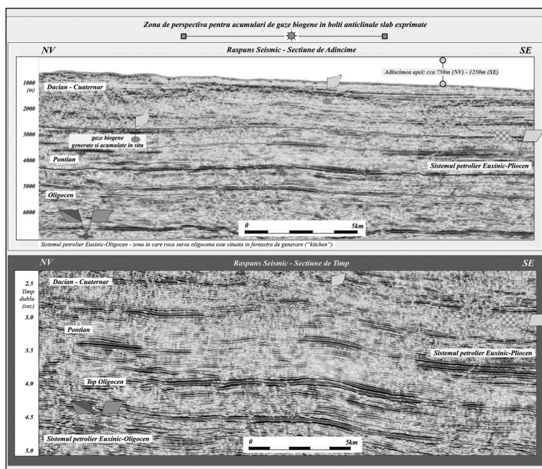
Figura 7. – Secțiune seismică de adâncime (a) și de timp (b) prezentând răspunsul seismic al zonelor de perspectivă pentru acumulări de gaze biogene cantonate în formațiuni pliocene situate în sectorul cu apă de mare adâncime al Depresiunii Histria. Capcanele subtile sunt reprezentate prin structuri de drapare a morfostructurilor terțiare, de tipul anticlinalelor de compactare slab exprimate și cu rază mare de curbură (sursă: Morariu, 2020; Total-FinaElf, 2002).
