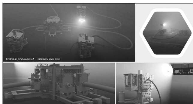
Figura 14. – Prezentare schematică a centrului de foraj submarin în ape de mare adâncime, ce va fi dezvoltat pentru valorificarea resurselor comerciale de gaze naturale din descoperirea Domino (colaj original de fotografii din arhiva ExxonMobil, OMV Petrom, 2021).
