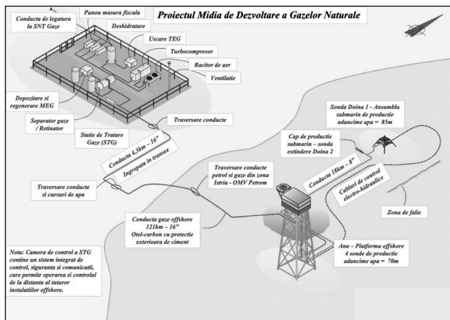
Figura 9. – Prezentare schematică a planului de dezvoltare pentru punerea în producție a acumulărilor de gaze naturale offshore Ana și Doina – Proiectul de Dezvoltare Gaze Midia (MGD) – realizat în prezent de compania Black Sea Oil and Gas (BSOG) – în calitate de Operator și Titular al Acordului Petrolier pentru Perimetrul XV Midia. Antreprenorul general pentru lucrările de execuție a Proiectului MGD este compania românească Grup Servicii Petroliere – GSP (cu modificări, după BSOG – Xodus FEED, 2017; BSOG – ESIA, 2020).
