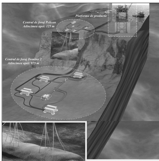
Figura 13. – Prezentare schematică a conceptului de dezvoltare a acumulărilor de gaze naturale din sectorul offshore cu apă adâncă – perimetrul Neptun Deep.
