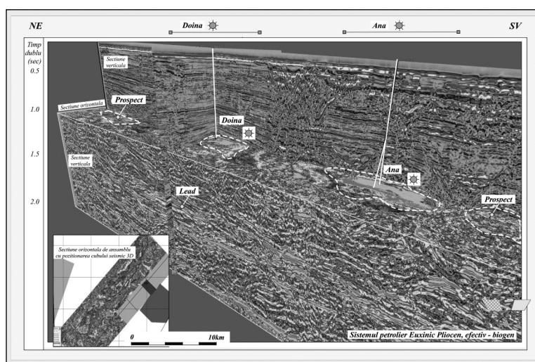
Figura 6. – Cub seismic 3D ilustrând cu ajutorul secțiunilor de timp verticale și orizontale geometria capcanelor subtile de pe aliniamentul productiv cu gaze biogene Doina – Ana, care reprezintă o terasă structurală dezvoltată în compartimentul ridicat al unei falii de creștere, precum și a altor zone de perspectivă pentru explorare în extindere a zonelor productive (cu modificări, după Morariu, 2020; Sterling Resources Plc, 2014).
