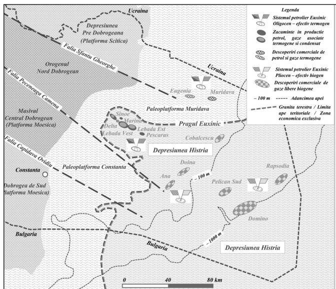
Figura 3 – Prezentare schematică a unităților structurale care intră în alcătuirea platoului continental românesc – sectorul de vest al Mării Negre – și a distribuției acumulărilor de hidrocarburi (cu modificări, după Constantinescu și Anastasiu, 2019; Morariu, 2020).
