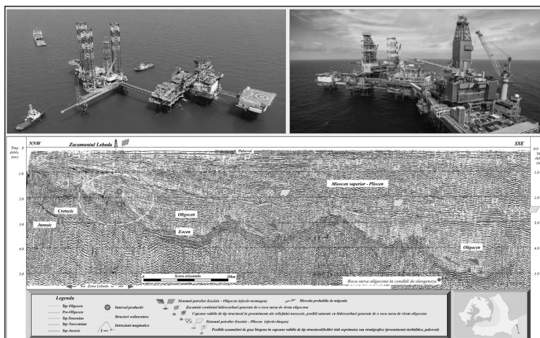
Figura 5. – Depresiunea Histria – Secțiune seismică regională ilustrând formarea acumulărilor de petrol și gaze de pe aliniamentul productiv Lebăda – Sistemul petrolifer Euxinic termogen (cu modificări, după Morariu, 2020).
