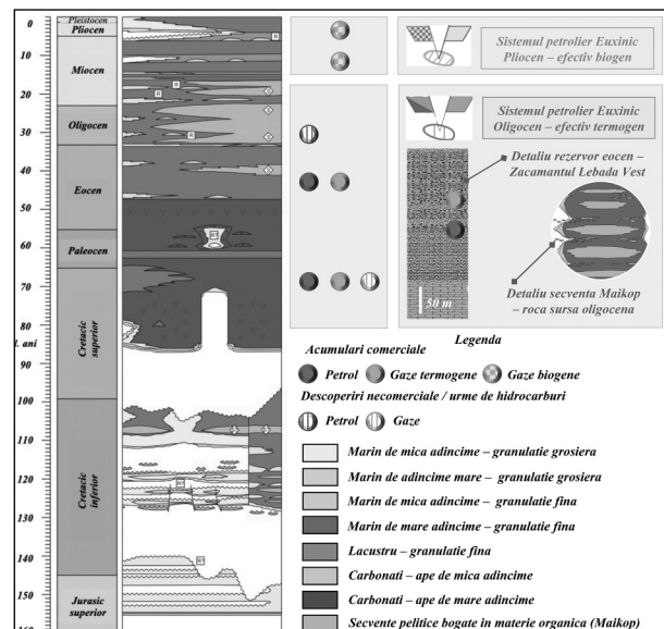
Figura 4 – Coloană chronostratigrafică simplificată a formațiunilor sedimentare din Depresiunea Histria cu precizarea sistemelor petrolifere efective și a principalelor ocurențe de hidrocarburi (cu modificări, după Simmons et al, 2018; Morariu, 2020).
