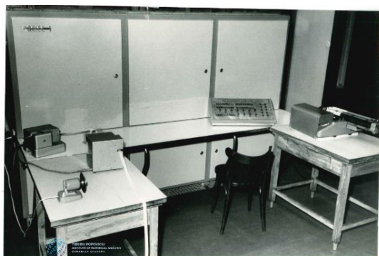
Figura 2. Calculatorul DACICC-1 în configurație complete.
