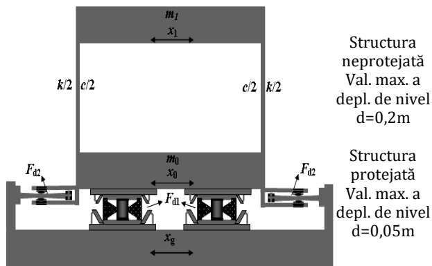
Figura 3. Reprezentarea schematică a structurii protejată seismic cu DISCON și DAICON.
