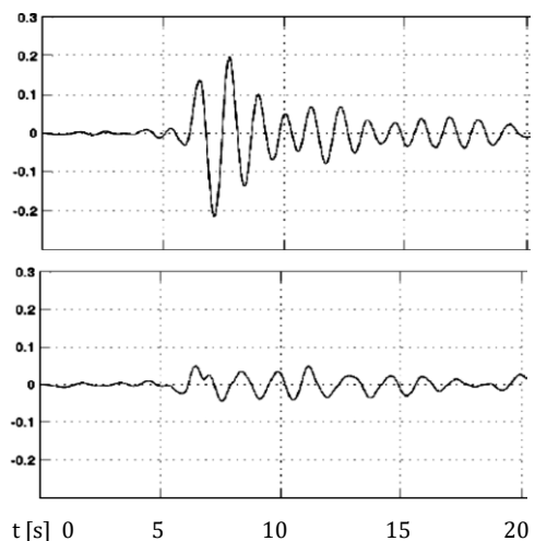
Figura 4. Analiza comparativă a deplasărilor de nivel la cutremurul Vrancea 77 a structurii protejate și neprotejate.
