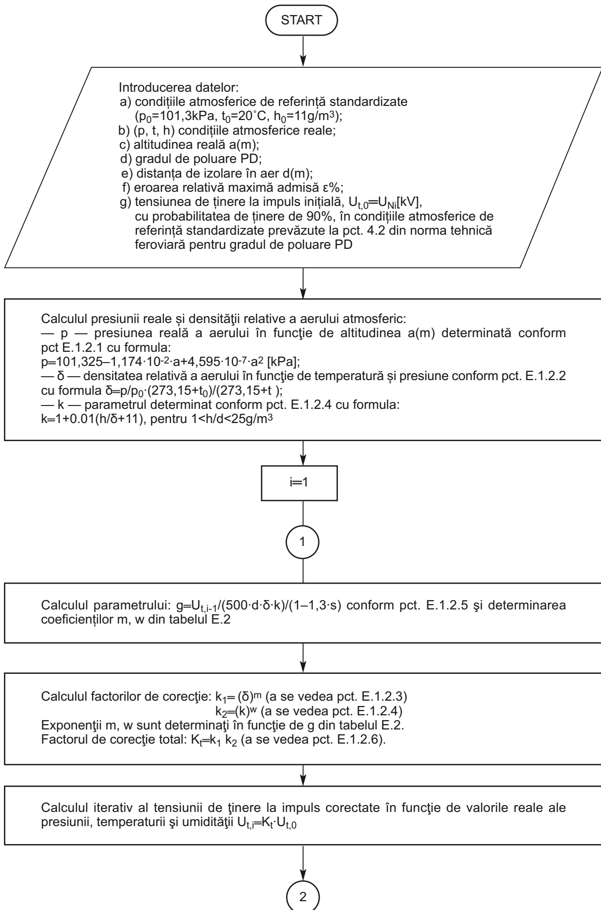
Figura E.1 — Schema logică a calculului privind determinarea și aplicarea factorilor de corecție de presiune, temperatură și umiditate în calculul tensiunii de ținere la impuls în condiții atmosferice reale
