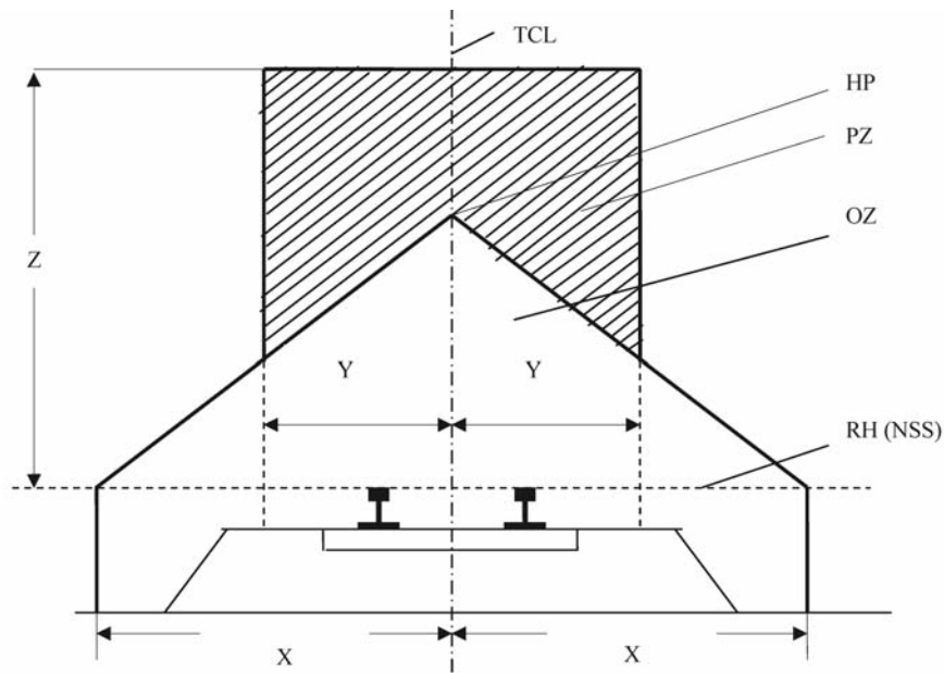
Figura 2*) — Zona liniei de contact aeriene și zona pantograf
